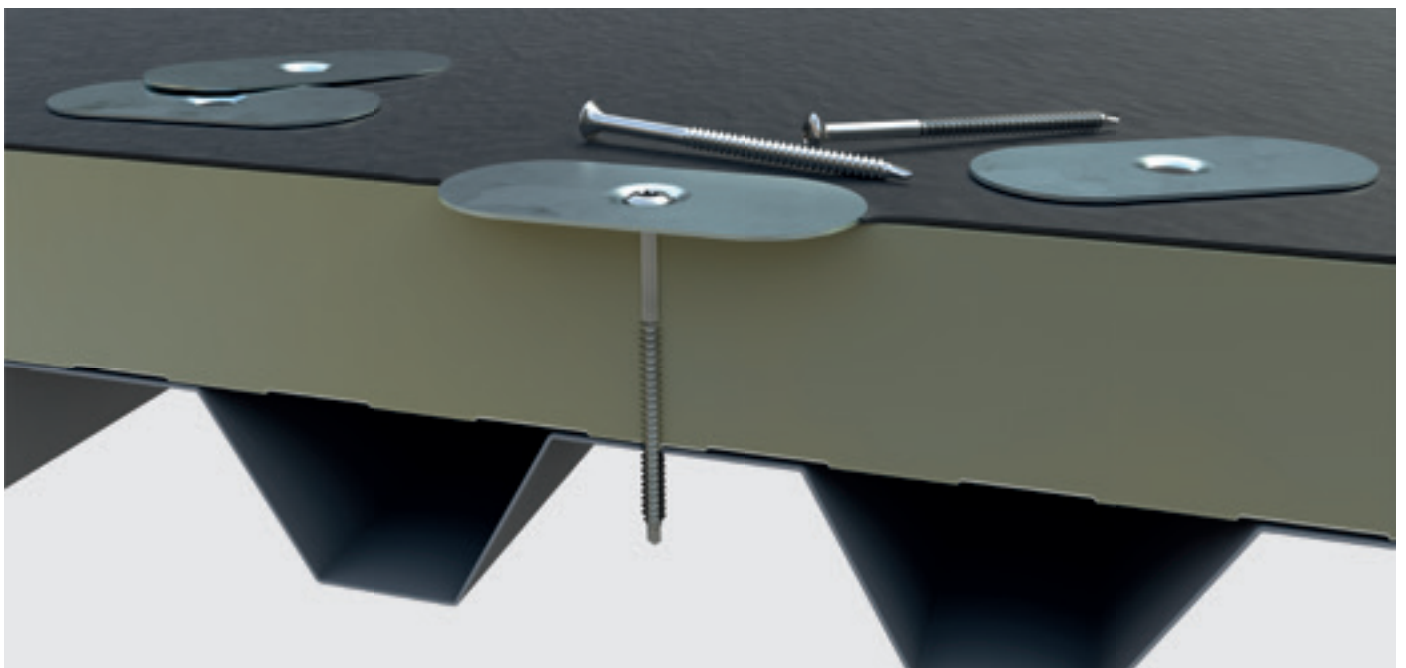
Befestigung der Flachdachdämmung mittels Trompetenkopfschraube und Halteteller (Der Halteteller ist nicht im Lieferumfang enthalten).
