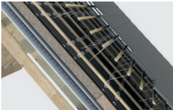
Aufdachdämmung an einem Schrägdach mittels Topduo Dachbauschraube.
