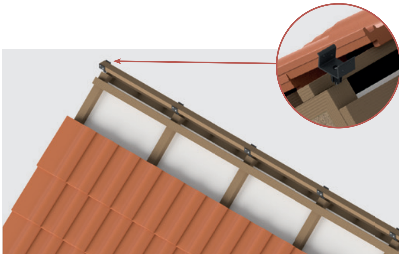
Montage des Grat- und Firstlattenhalters 50 im Sparren.
