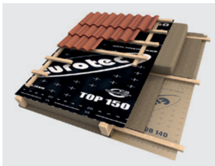
Beispielhafte Dachkonstruktion mit der verbauten Eurotec Unterdeck- / Unterspannbahn Top 150.
