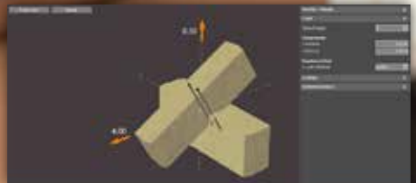
Modul für Sparren-Pfetten-Verbindungen mit Panelwistec- und KonstruX-Schrauben.
