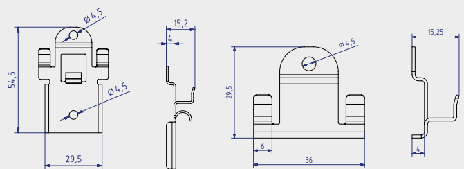
Fassadenclip-Rhombus
