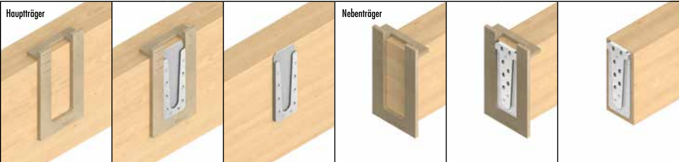
Aufgesetzte Montage des Magnus Einhängeverbinders: links auf Hauptträger, rechts auf Nebenträger
