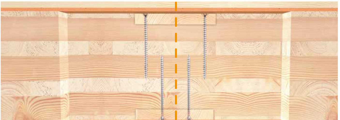
KonstruX en unión de forjado con ranura superior e inferior
