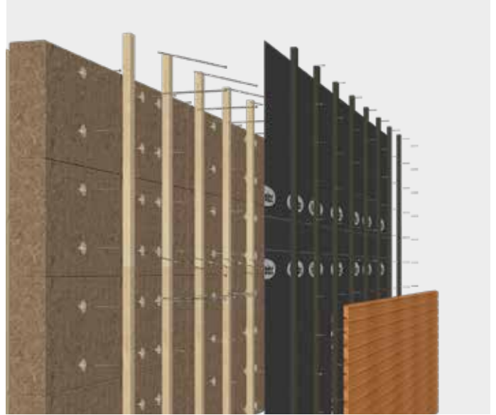
Fijación de fachada mediante listones de madera dispuestos vertical
