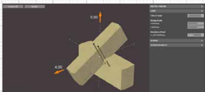
Módulo para conexiones entre cabrios y correas con Panelwistec y KonstruX
