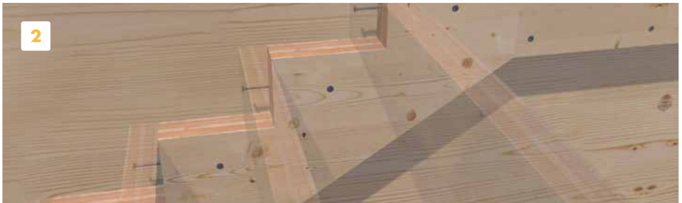
Mise en place de la finition de marche à l'avant du support de marche.
