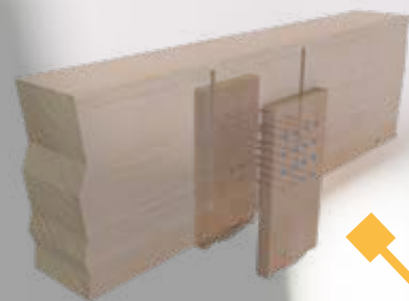
ASSEMBLAGE LATÉRAL À COUVREJOINTS
