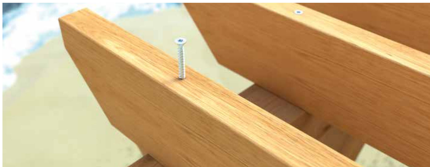
KonstruX con testa svasata in acciaio inossidabile A4: ideale per collegamenti legno-legno in aree urbane e industriali inquinate > 0,25 km dalla costa.
