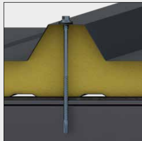
Befestigung im Obergurt ohne Kalotte
