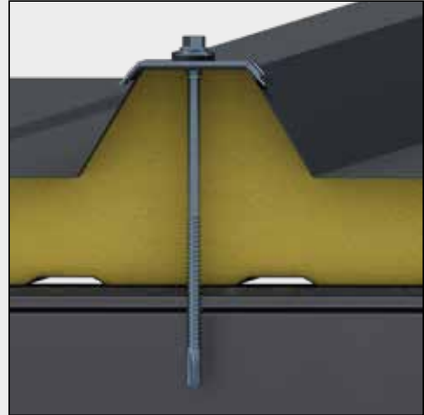
Befestigung im Obergurt mit Kalotte
