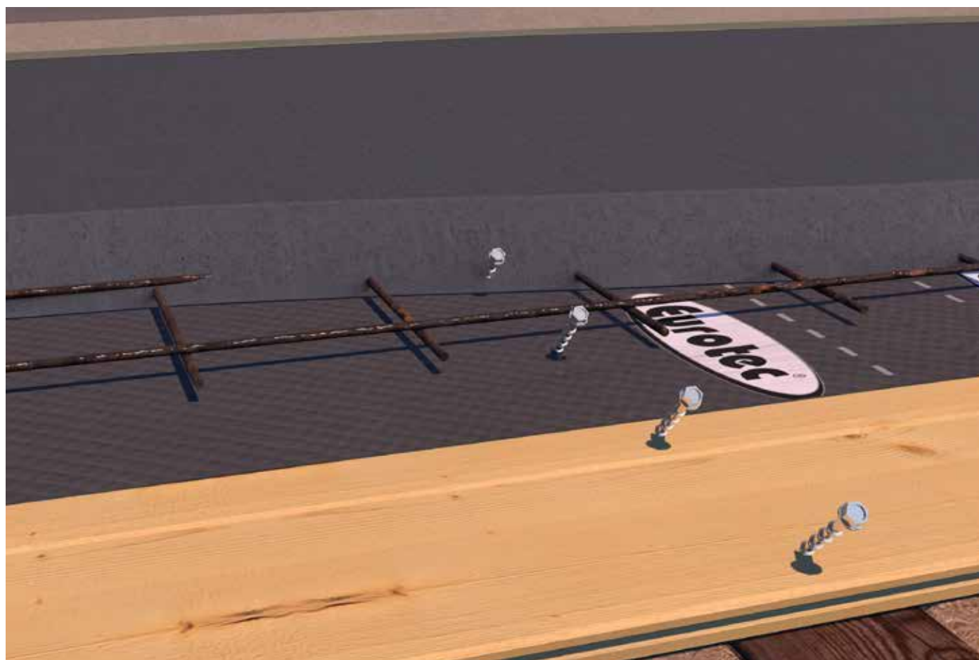
Trittschallentkopplung und Estrich auf der HBV-Decke
