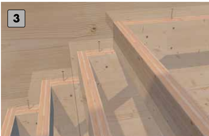
Stufen oben auf der Stufenauflage anbringen.
