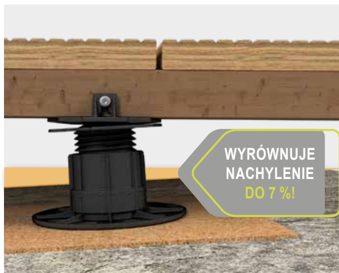
Przykład zastosowania: drewniane konstrukcje nośne
