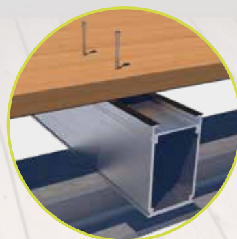
Zamocowanie widoczne przez profilowy wkręt samowiercący
