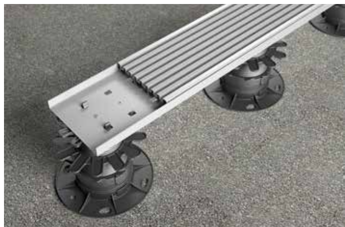
DrainTec Base w połączeniu z kratownicą odpływową DrainTec i nóżkami regulacyjnymi PRO z adapterem zatrzaskowym.
