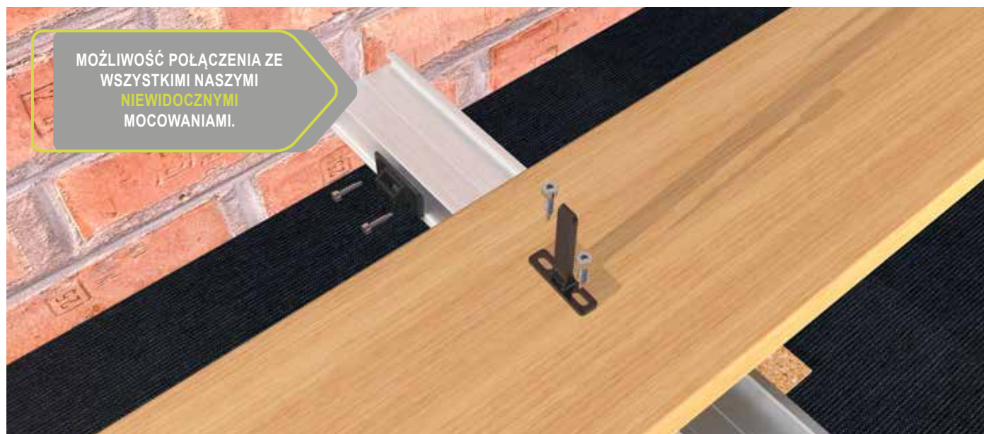
Wtyk mocuje się pod deską, a następnie można go zatrzasknąć w uchwycie.
