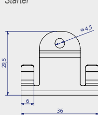
Klips fasadowy Rhombus Starter
