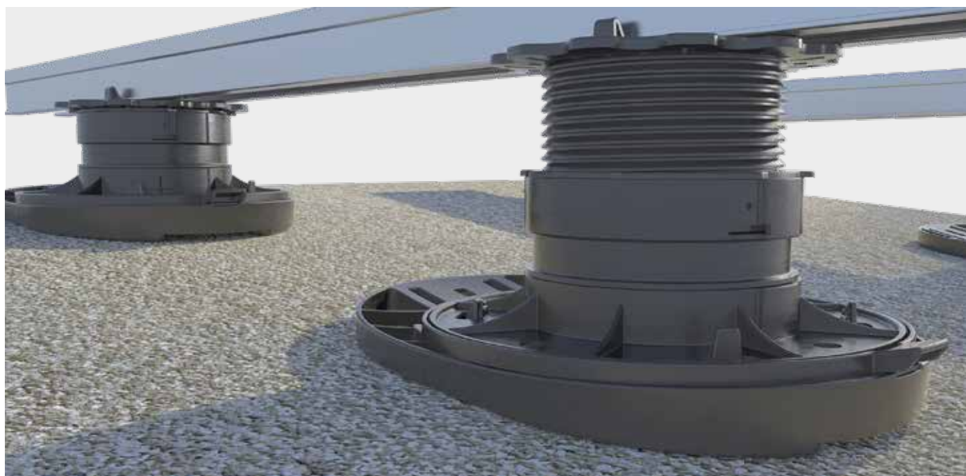
Wyrównanie spadku za pomocą Nivello 2.0.
