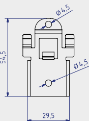
Klips fasadowy-Rhombus
