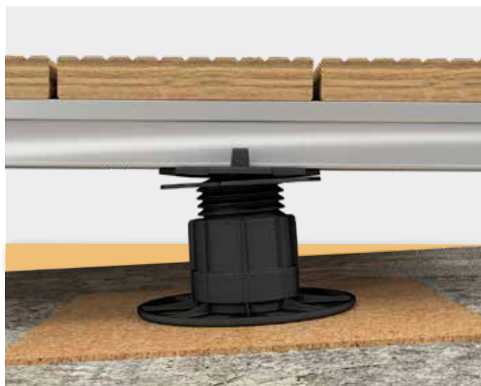
Przykład zastosowania: aluminiowe konstrukcje nośne
