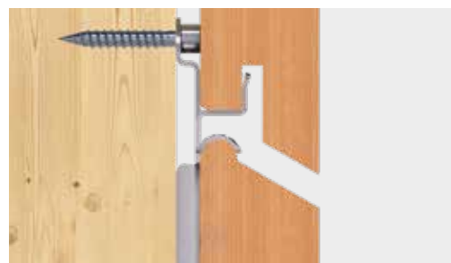
Wandanschluss mit Fassadenclip-Rhombus
