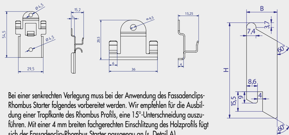
Fassadenclip-Rhombus
