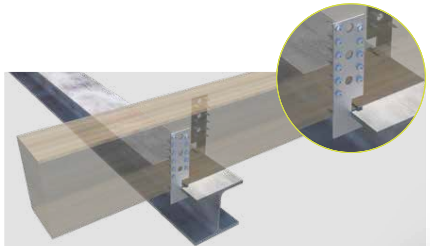
T-Träger Anker in Verbindung mit einem T-Träger.
