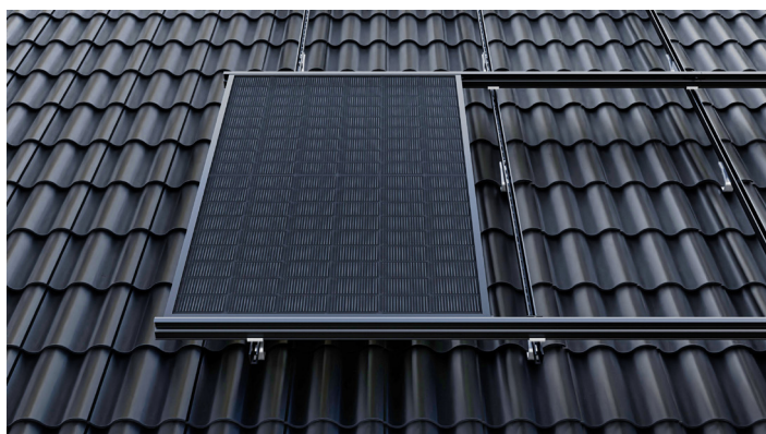
SCHRITT 22: Fertig eingesetztes Solarmodul
