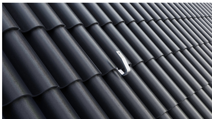
SCHRITT 6: Dachhaken LayTec im montierten Zustand.
