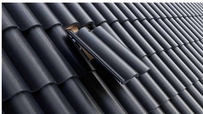
SCHRITT 1: Im ersten Schritt wird die Dachpfanne vom Dach gelöst.
