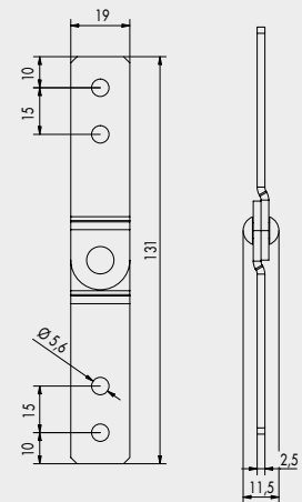
Articulación de 90° TERRA
