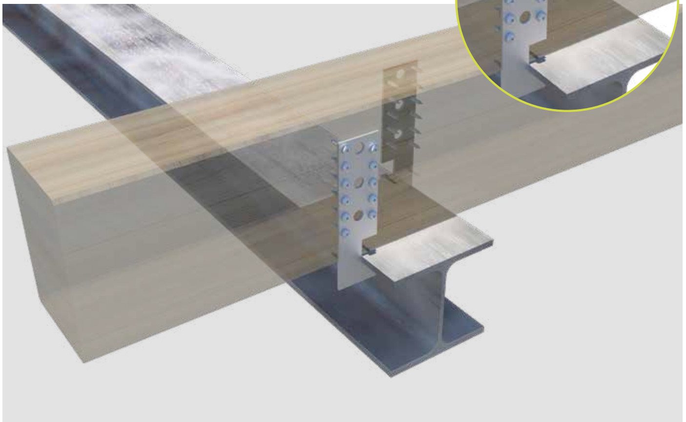
Anclaje para perfiles T usado en una viga laminada doble T.
