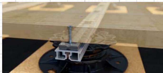
Ejemplo de aplicación Perfil de aluminio TERRA H15
