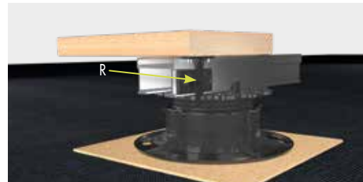
Fijando una tabla de madera al sistema de perfilera de aluminio EVO utilizando el Conector a presión (R).
