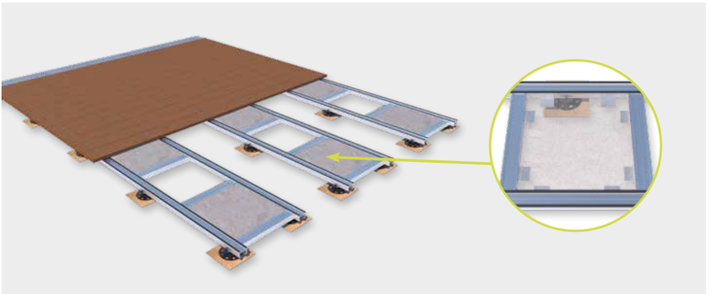
Sujeción contra la succión del viento en terrazas de madera con el uso de losetas apoyadas en las escuadra de sobrecarga
