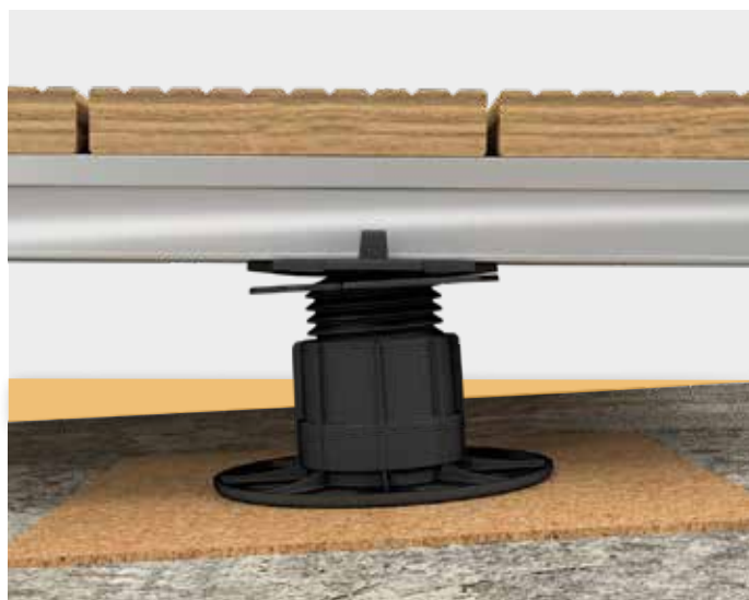
Ejemplo de aplicación en subestructura de aluminio
