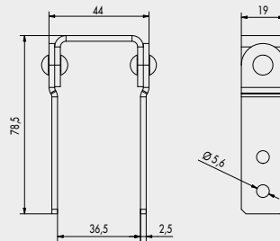
Articulación de 90° TERRA
