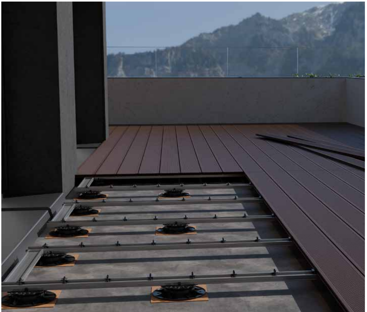
Subestructura con plots regulable PRO, adaptador click 60, sistema de perfilería de aluminio EVO y grapa Twin
