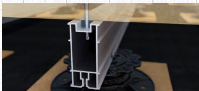
Ejemplo de aplicación Perfil de aluminio TERRA H85
