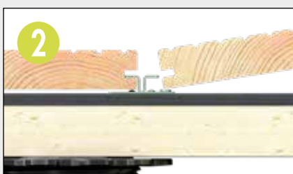
Fijación de la madera en el clip de terraza RI4 para que ambos dientes queden junto a la ranura de la tabla.
