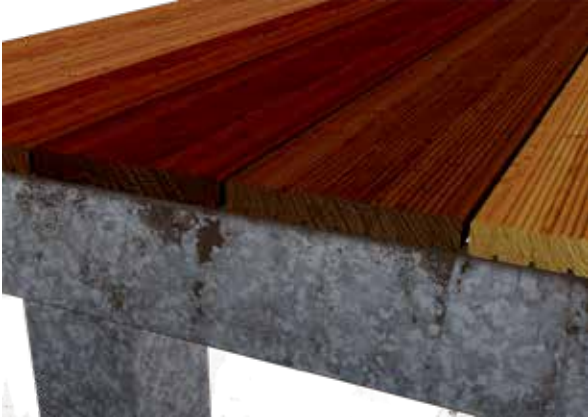
Auswaschungen aus Bangkirai, die sich nur durch eine konstruktive Lösung, z. B. Abtropfblech, verhindern lassen
