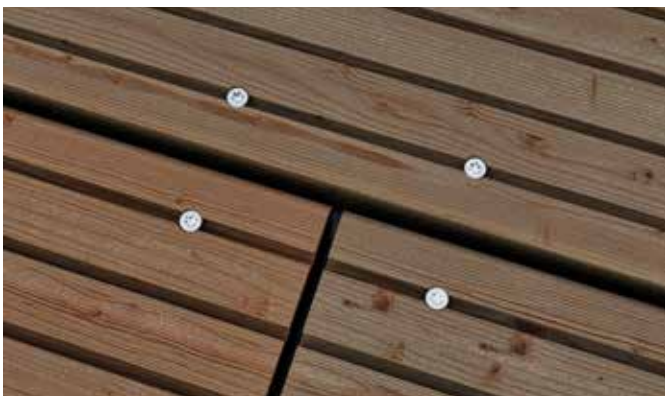
Verschraubung im Nutengrund: Bei Geh-, Fahrweg und Brückenbelägen Stand der Technik
